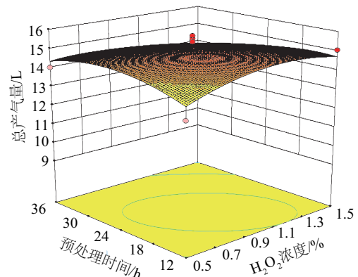
图3 预处理时间与 H_2O_2 浓度响应面图
