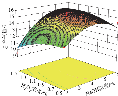
图2 H_2O_2 浓度与 NaOH 浓度响应面图
